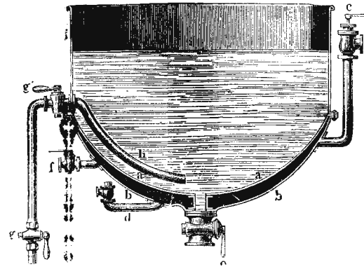
3. Дефекационный котель.
