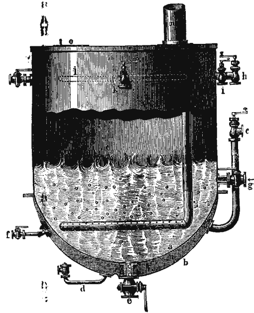
4. Сатурационный котель.
