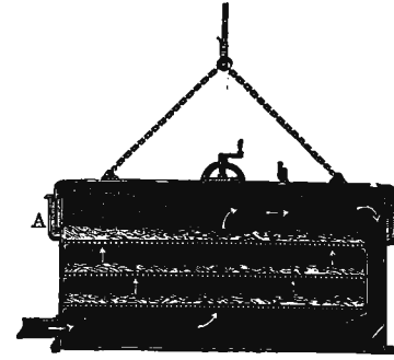
6. Разрывъ очистительнаго ящика.
