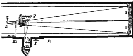
Рис. 1. Ресфлекторъ Ньютона.
