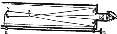
Рис. 3. Ресфлекторъ Грегори.
