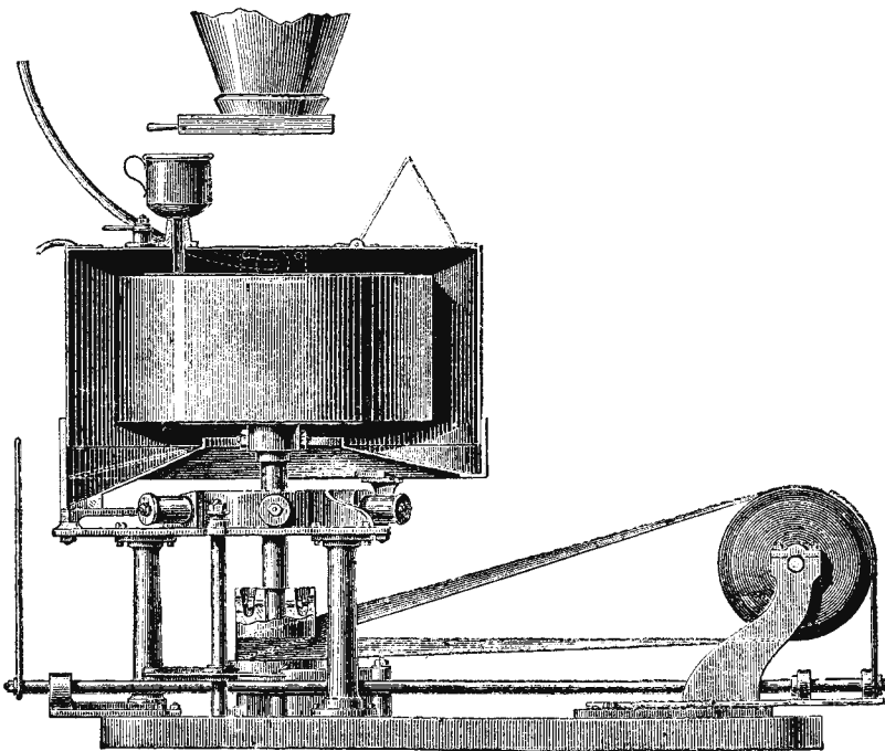
9. Центрофуга.
