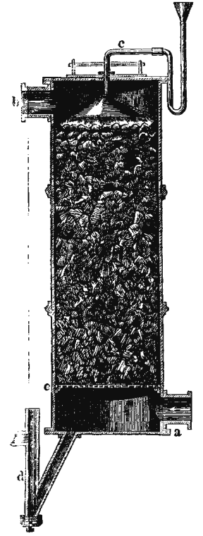
4. Скрубберъ.
