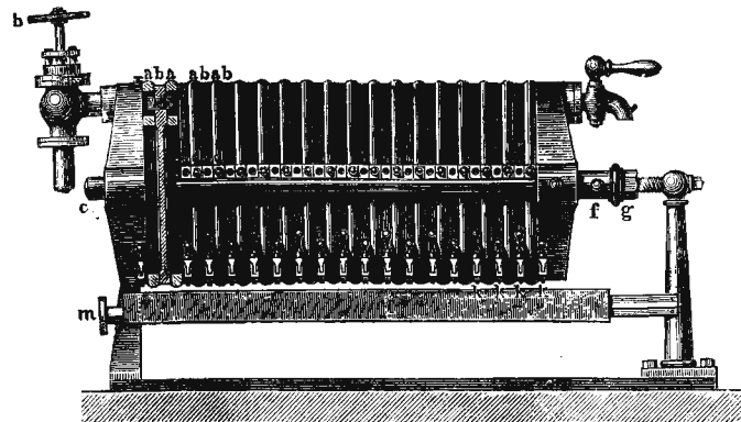
5. Фильтрпрессъ.
