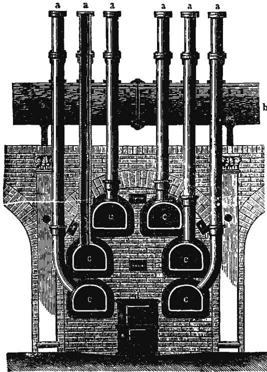
1. Реторты.
