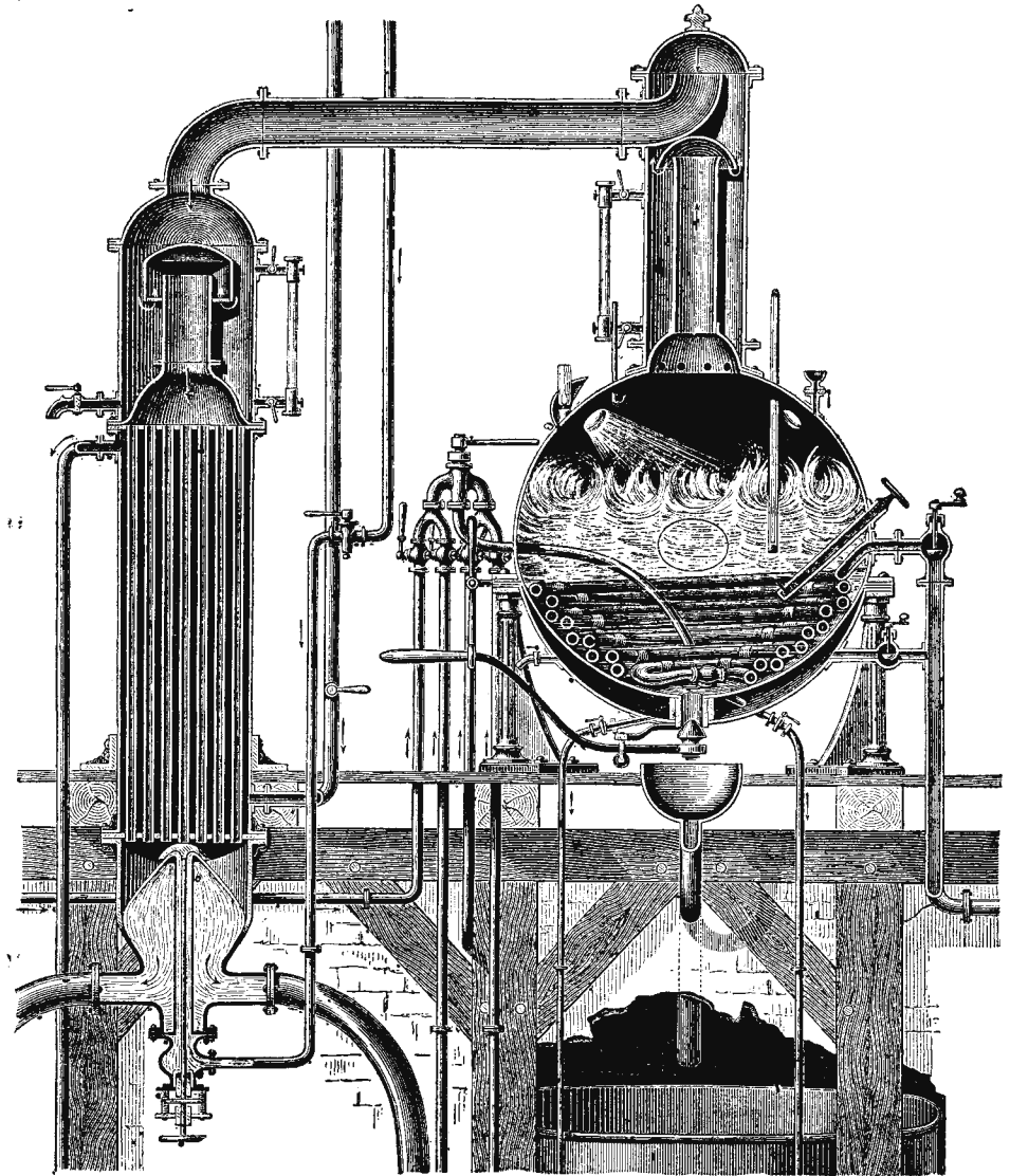
8. Вакуум-аппаратъ.
