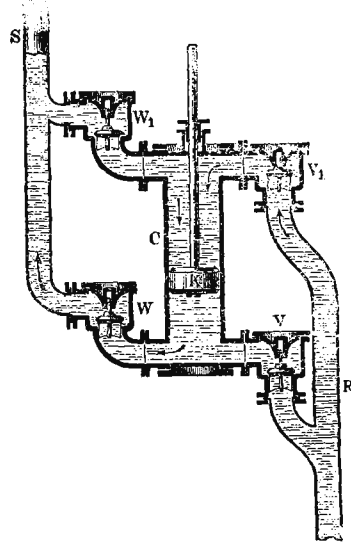
Насосъ. Рис. 2.
