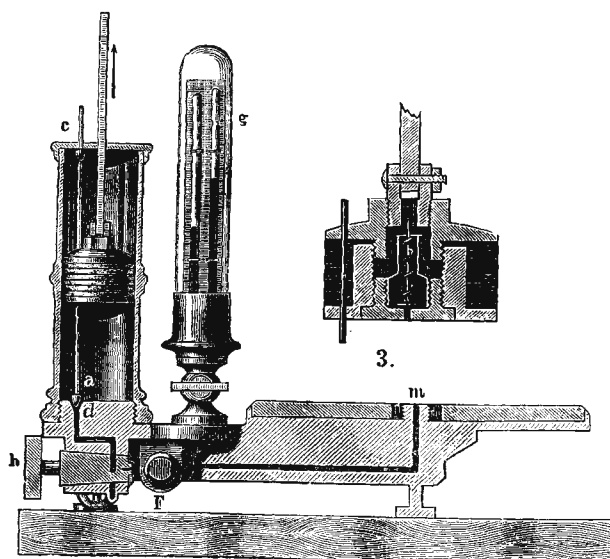
Черт. 2. Двухцилиндровая пневматическая машина в разрезе.
