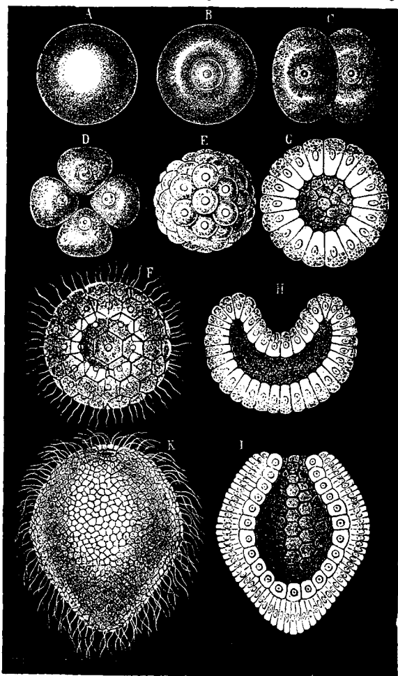
Стадии развития Monoxenia Darwinii (увелич.).
