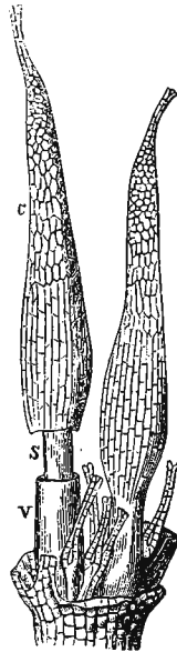
Мхи. Рис. 5. Женскій цвѣтокъ съ двумя спорогоніями.
