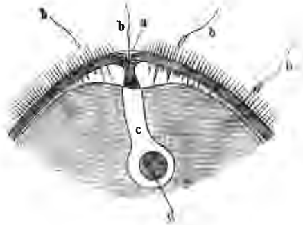
Рис. 2. Верхній отгѣзокъ яйца миноги (Pelomonon): а отверстие для прохода сѣмянныхъ нитей, „микрочипа“; б сѣмянный каналъ; с каналъ, по которому сѣмянная нить достигаетъ зародышка d.
