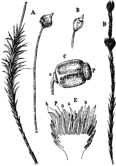
Мхи. Рис. 3. Цилиндрическій мохъ, Polytrichum commune . А женская особь въ капсулѣ, В и С капсула, D мужская особь, E мужской цвѣтокъ.
