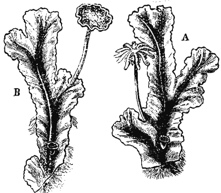
Мхи. Рис. 2. Marchanti Polymorpha . А женская особь съ плодоношеніемъ, В мужская особь съ плодоношеніемъ.
