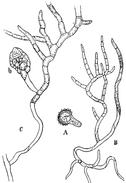
Мхи. Рис. 1. Проростающая спора и проростки листовыхъ мховъ. А спора, В и С проростки, Д зачатокъ стволика.
