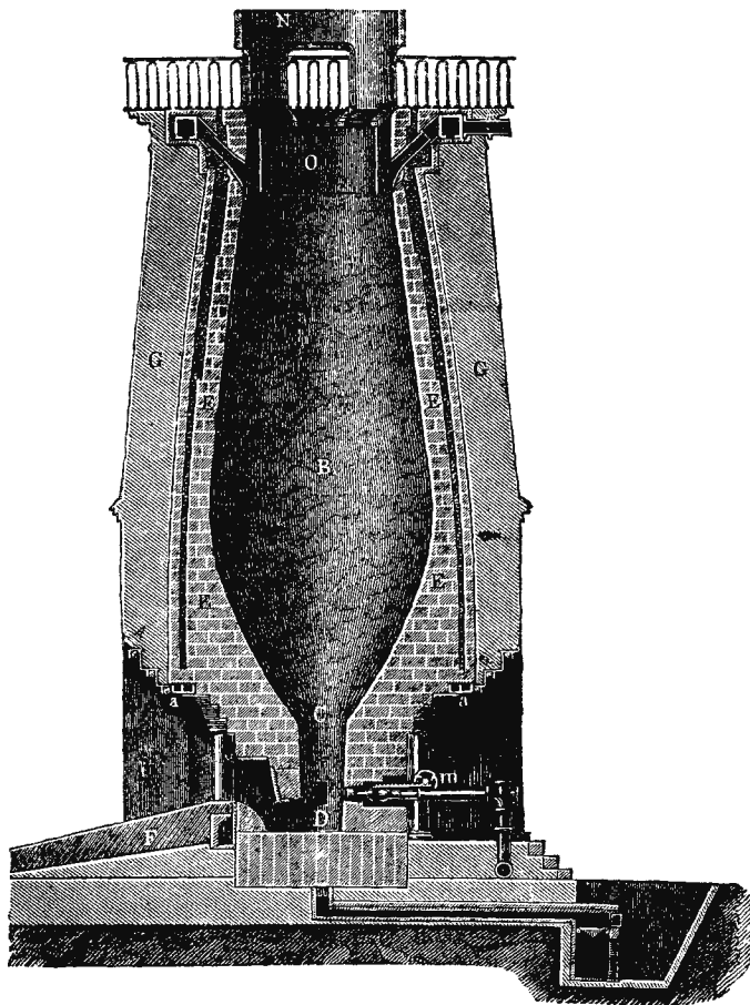
Доменная печь.
