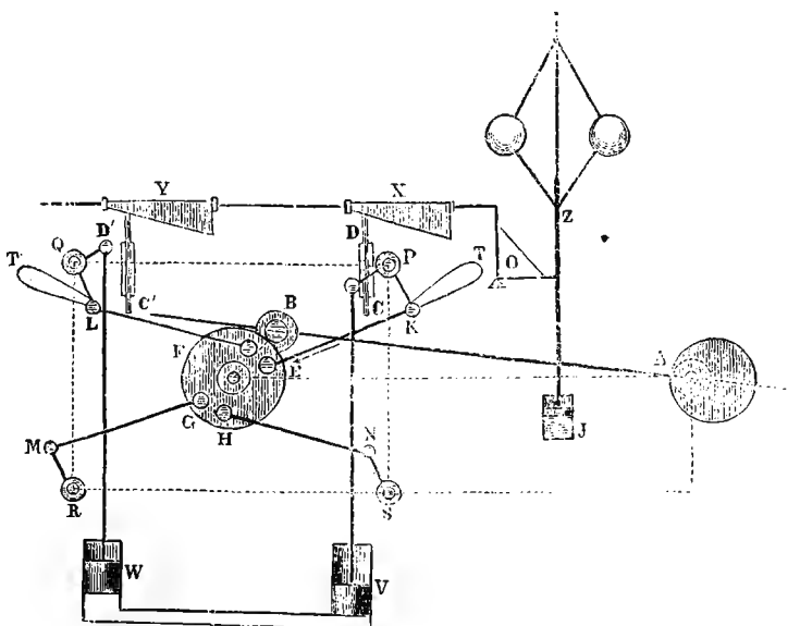
Схема парораспределительнаго механизма Корлиса.
