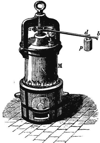
Папиновъ котель.
