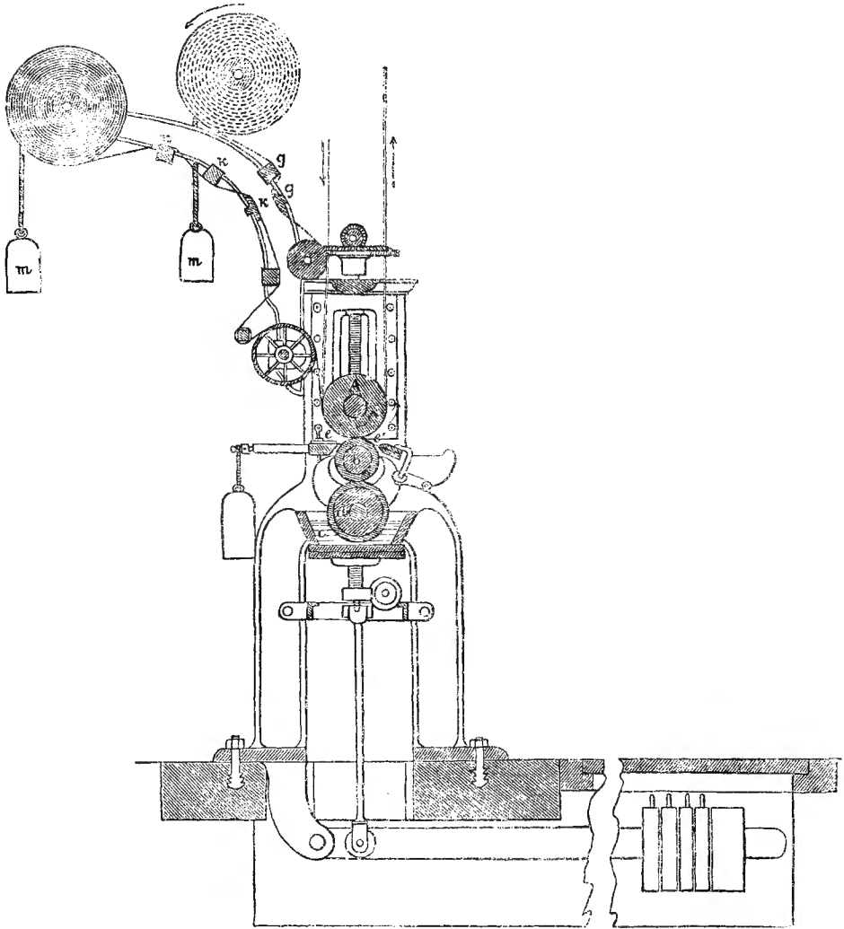
Набивная машина.
