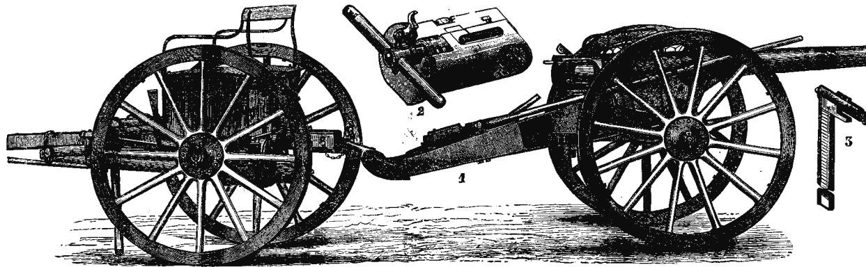
1) Полевая пушка (завода Круппа). 2) Клиновой затвор полевой пушки. 3) Прицѣлъ.
