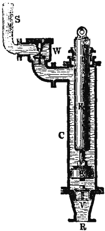
Насосъ Рис. 1.
