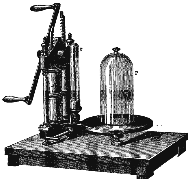
Черт. 1. Общий вид двухцилиндровой пневматической машины.
