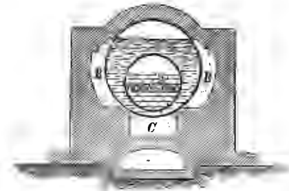
Корнваллійскій котель.
